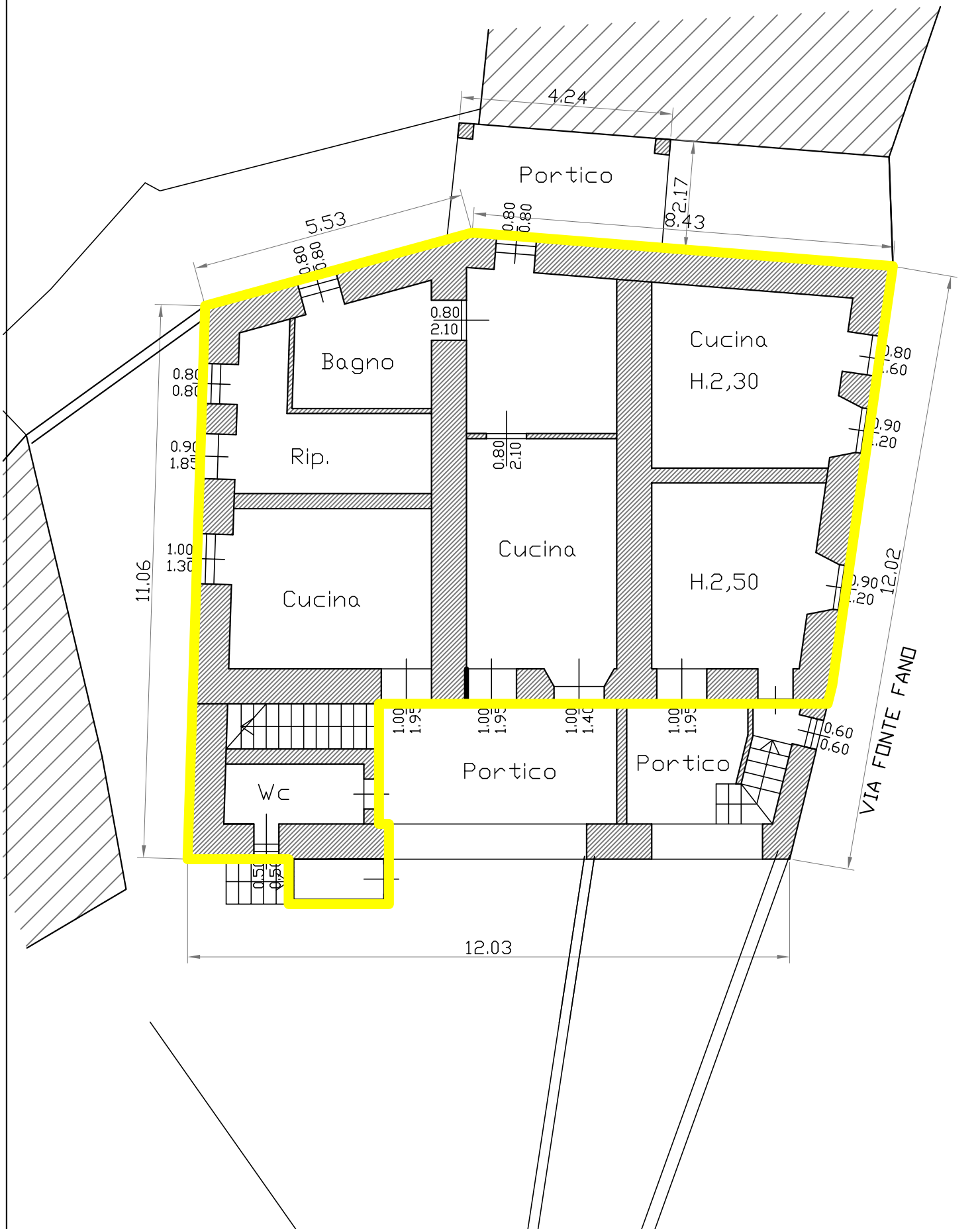
PIANTA PIANO TERRA SCALA 1:100 - SL MQ.131,50
