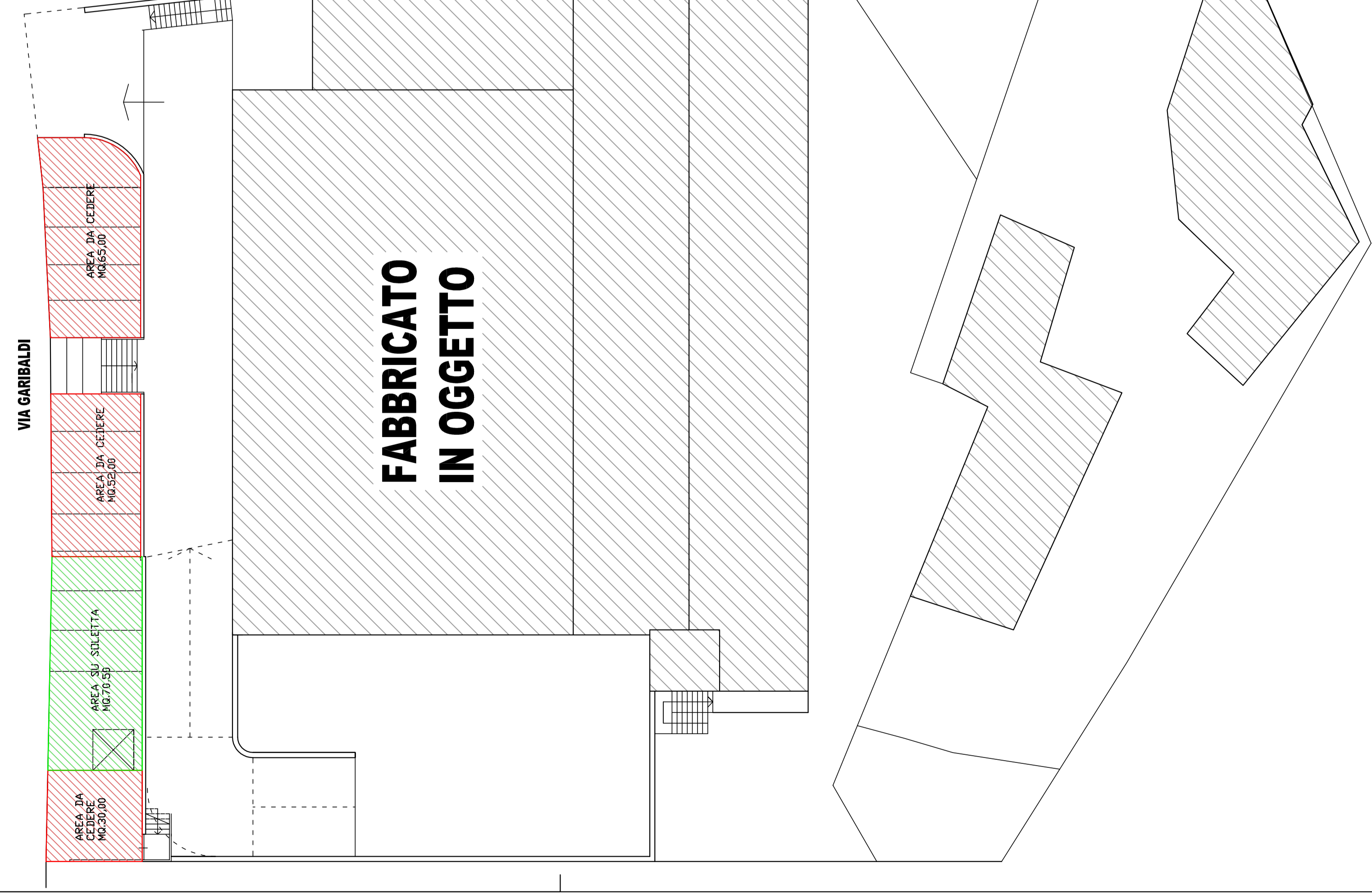
PLANIMETRIA GENERALE ESISTENTE SCALA 1:200
