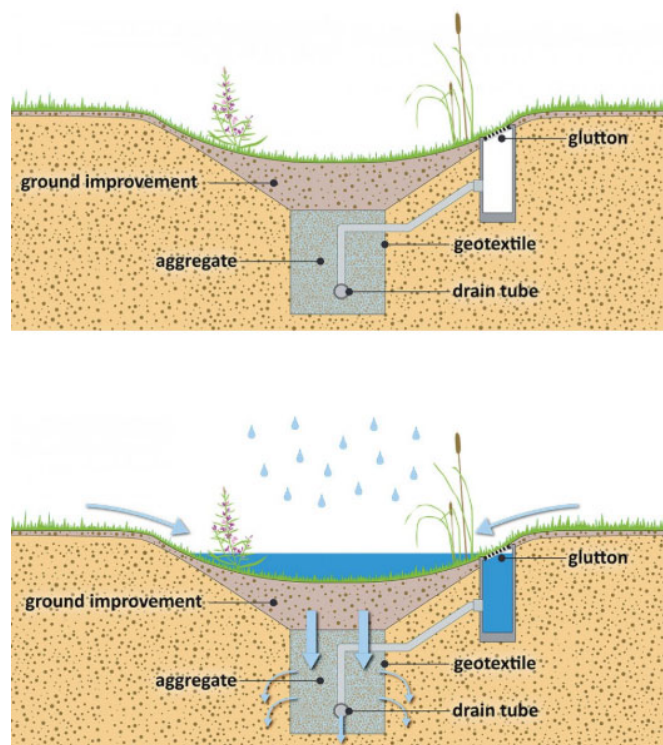
Figura 35. Schema tipo
