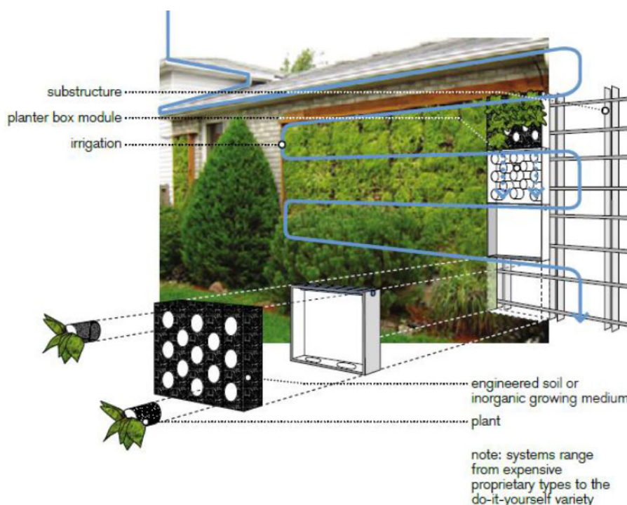
Figura 20. Esempio di struttura a Parete Verde
