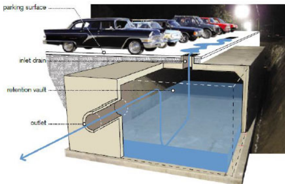
Figura 10. Schema esemplificativo
