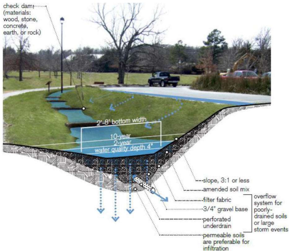
Figura 6. Schema tipo di fosso disperdente
